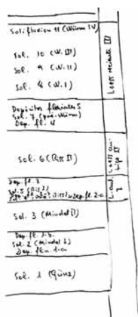
Esquema estratigráfico de Álvarez Blázquez onde se indican a evolución dos solos en función das diferentes etapas dos ciclos glaciares do sistema alpino. Arquivo Álvarez Blázquez.
