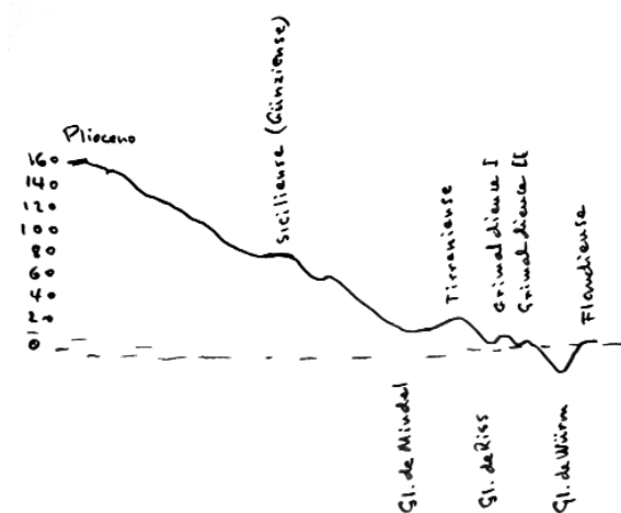
Debuxo de Álvarez Blázquez onde se representan os diversos episodios de transgresión/regresión mariñas (parte superior) e a súa relación cos ciclos glaciares alpinos (parte inferior) na bacia do río Miño. Arquivo Álvarez Blázquez.
