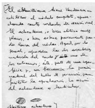
Texto original, escrito a bolígrafo, onde explica a diferenza entre o abbevilense e o achelense. Arquivo Álvarez Blázquez.
